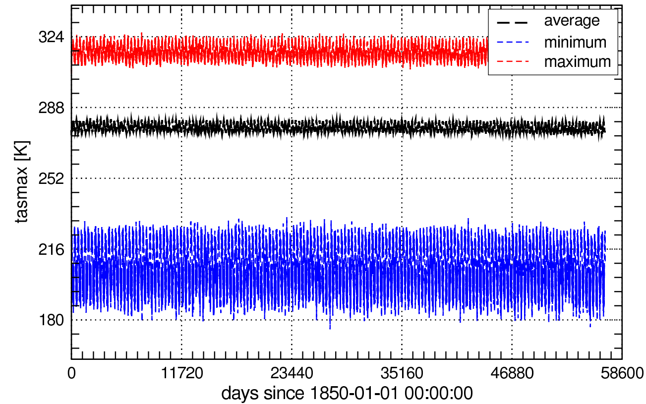
Global Values of tasmax_day
