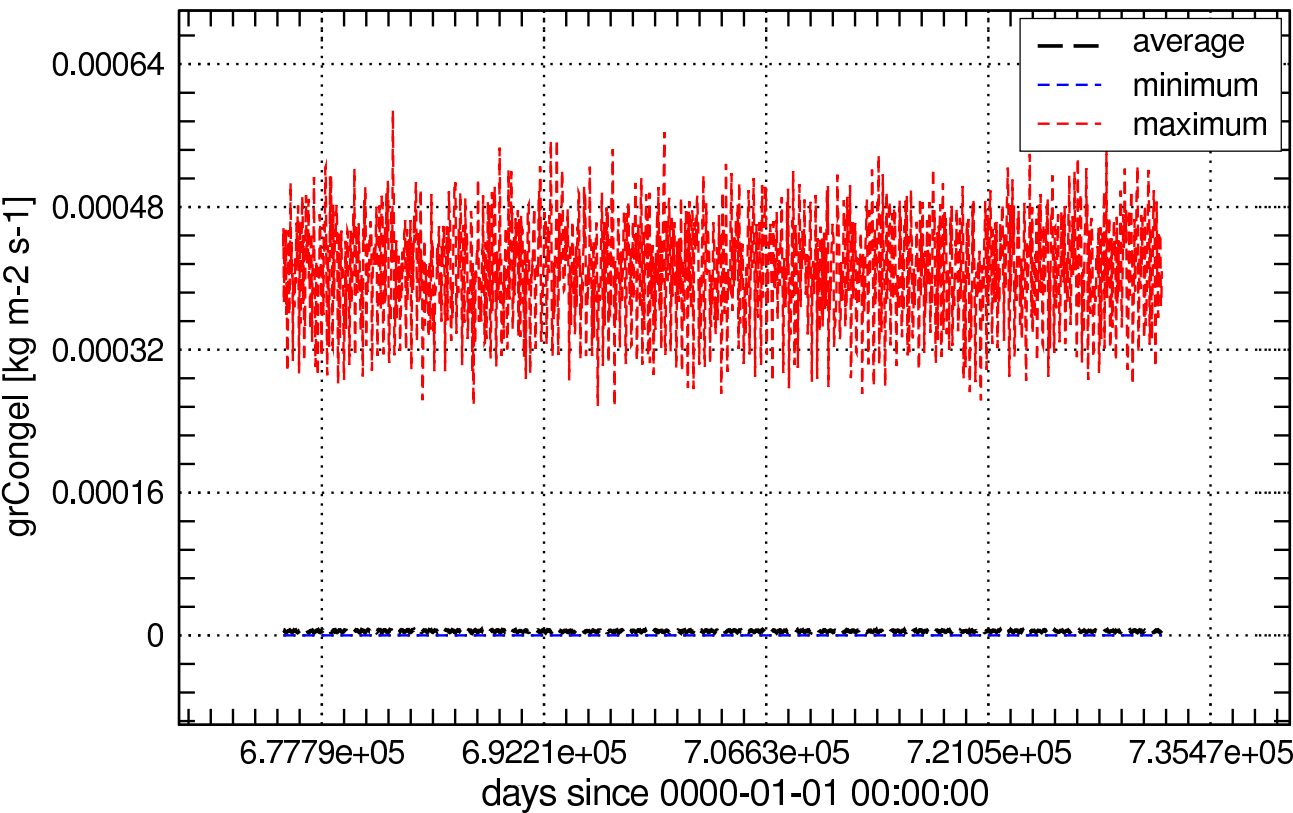
Global Values of grCongel_Olmon
