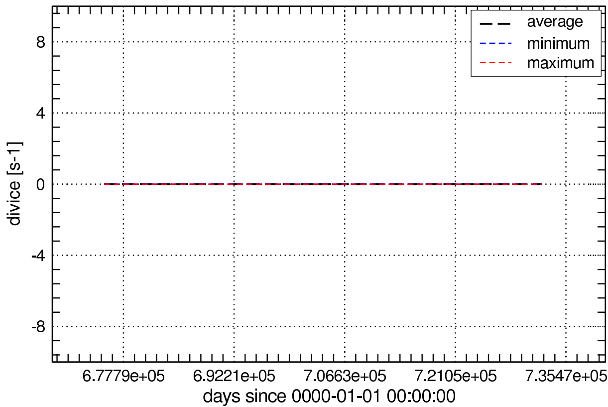
Global Values of divice_Olmon
