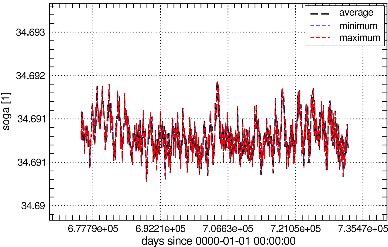
Global Values of sog a _Omon
